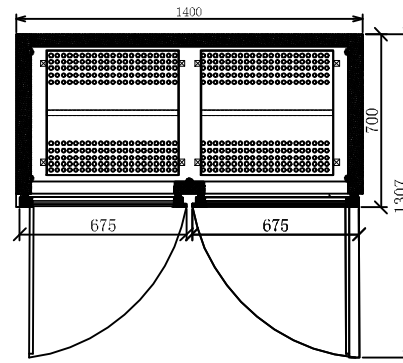
Top View 俯视图
